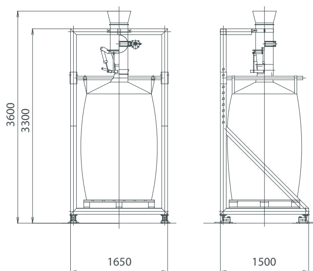
Particolari del sistema di sbattimento per prodotti a difficile scorrimento. Details of the bottom shaking system for difficult flowing products.
